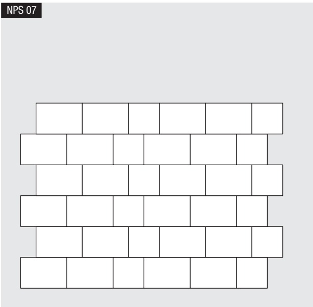
Gemischter Läuferverband – mit 2 Steinformaten
