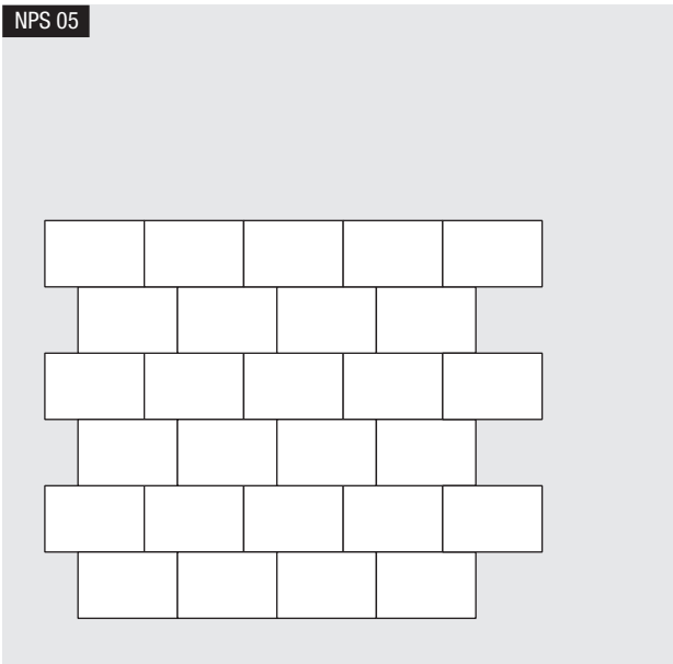
Läuferverband – mit 1 Steinformat / Drittelsteinversatz
